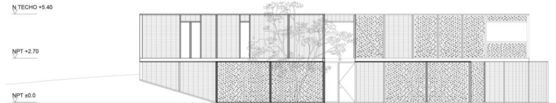
ELEVACIÓN NORTE
