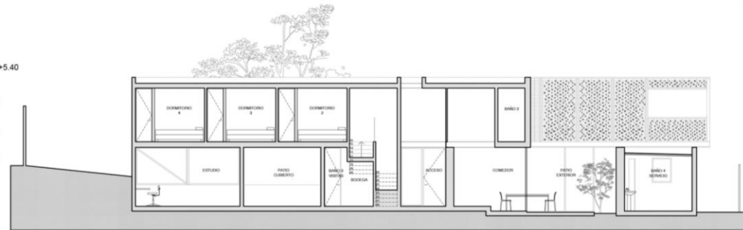
CORTE B-B'
