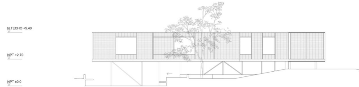
ELEVACIÓN ORIENTE
